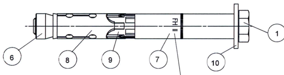
Sechskantschraubenversion S
